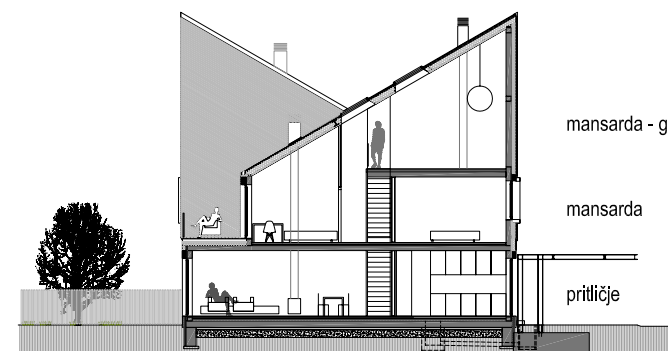
prečni prerez
