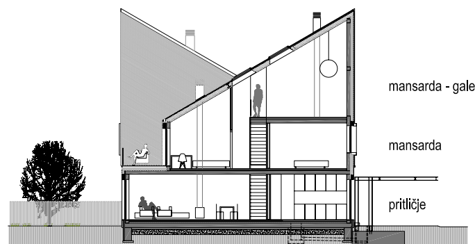
prečni prerez
