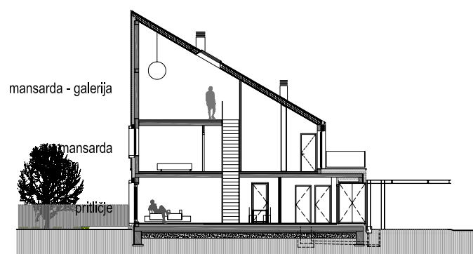
prečni prerez
