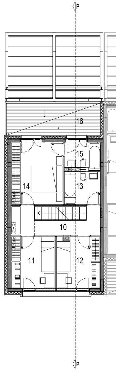
tloris mansarde
