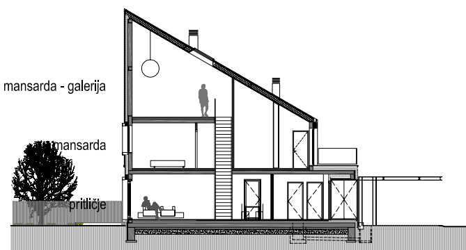
prečni prerez
