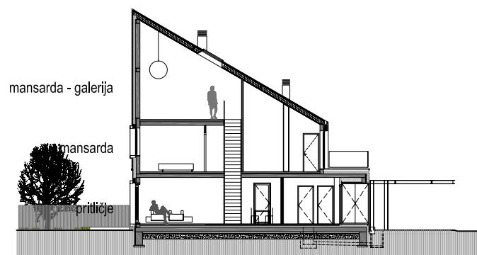
prečni prerez
