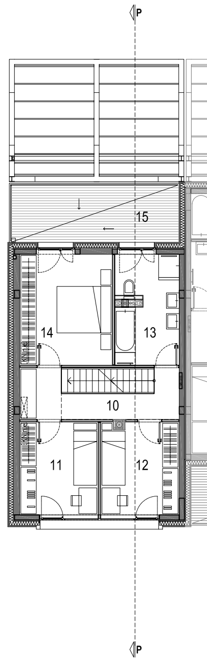
tloris mansarde
