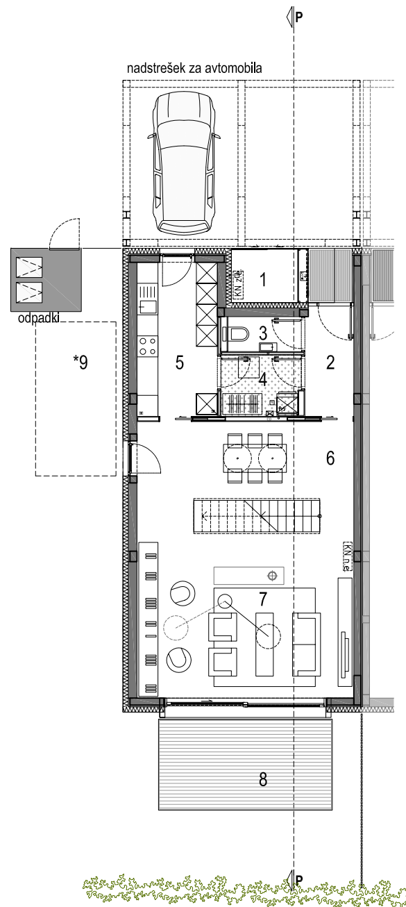
tloris pritičja
