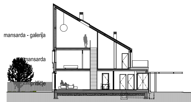
prečni prerez
