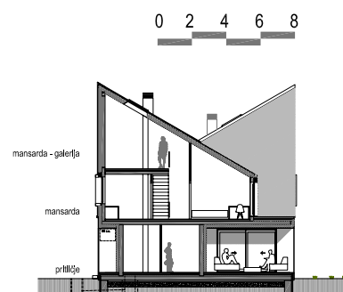
prečni prerez
