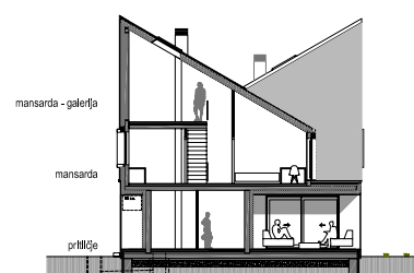
prečni prerez
