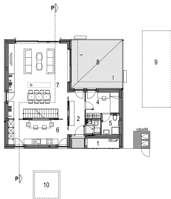
tloris pritličja
