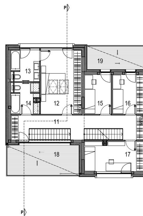
tloris mansarde
