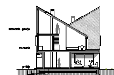
prečni prerez
