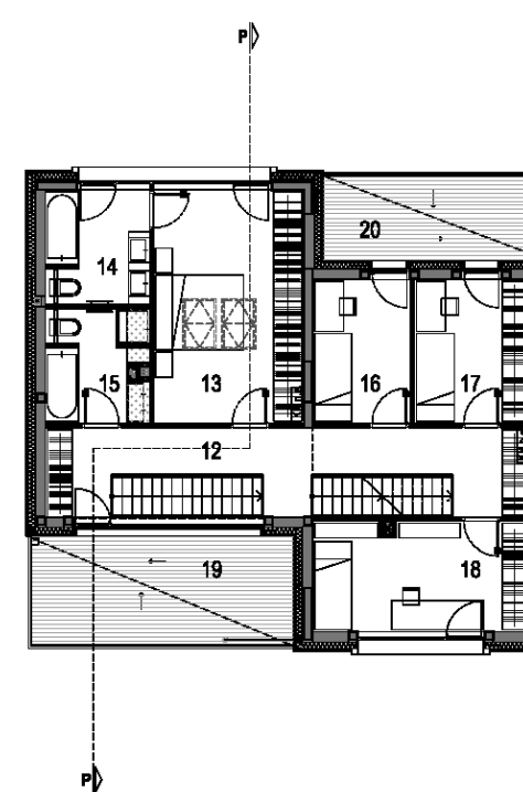
tloris mansarde
