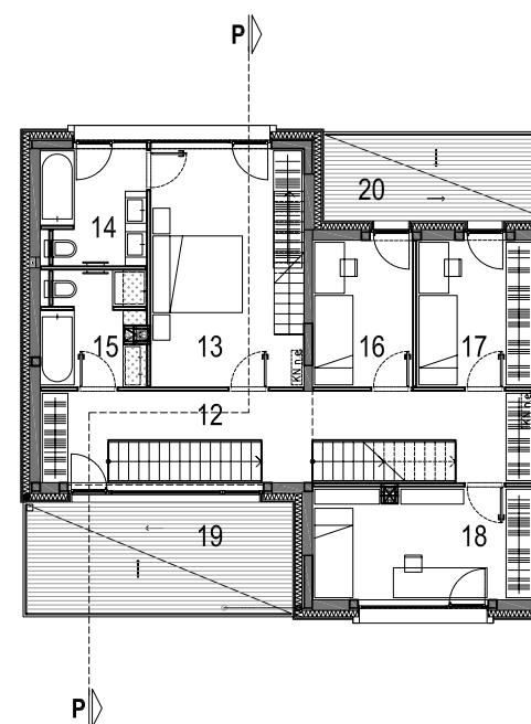
tloris mansarde
