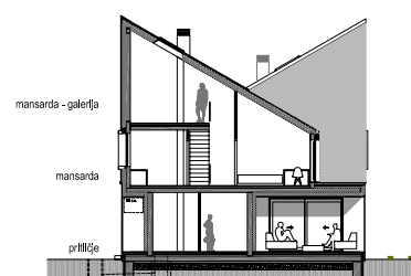
prečni prerez
